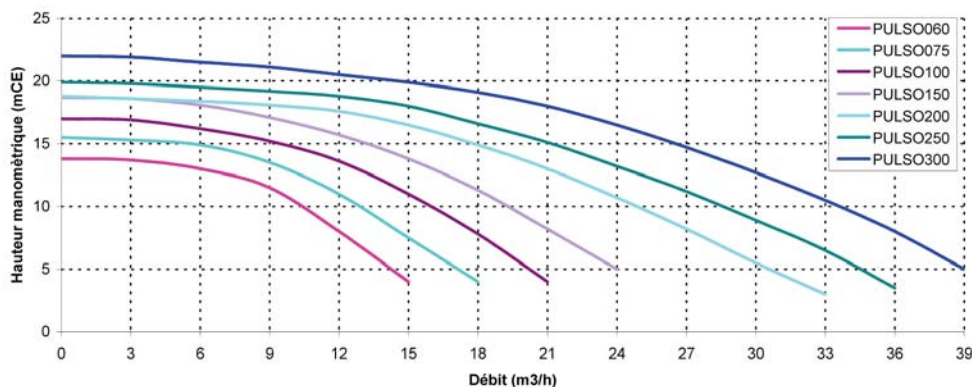
Courbes Hydrauliques PULSO 0,5 à 3CV
